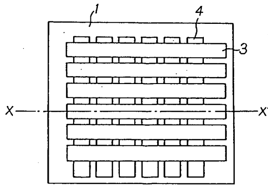
素子の平面図
